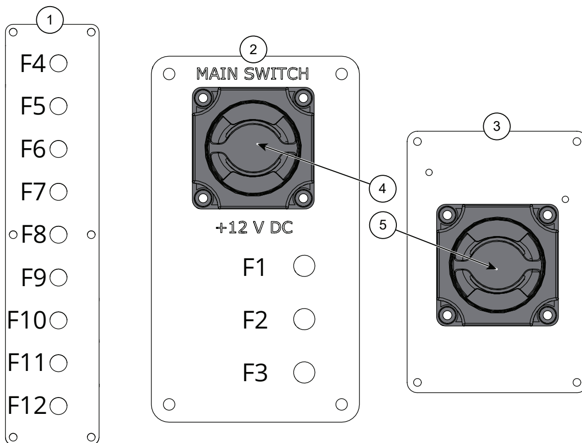
Figur 8.1 Hovedbrytere og sikringspaneler i Buster XL/XXL
