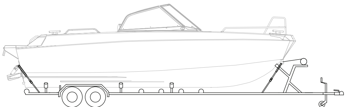
Figur 12.1 Tilhengertransport av Buster XL/XXL
