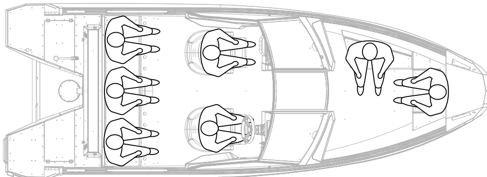
Figur 4.1 Buster XL seter for maksimalt sju (7) passasjerer
