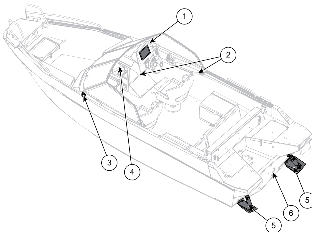
Figur 8.4 Elektrisk utstyr i Buster XL/XXL
