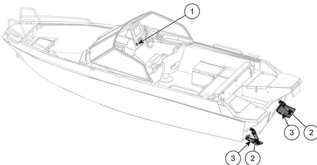
Figur 5.4 Komponenter i trimsystemet i Buster XL/XXL
