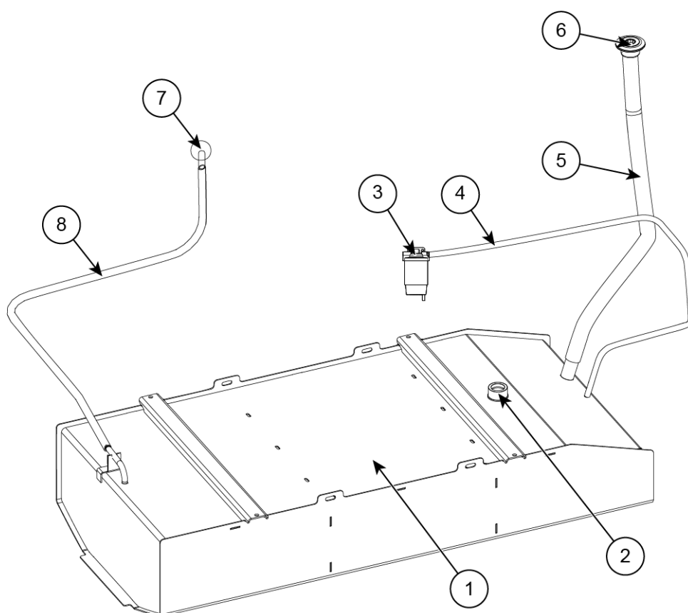
Figur 6.1 Drivstoffsystem
