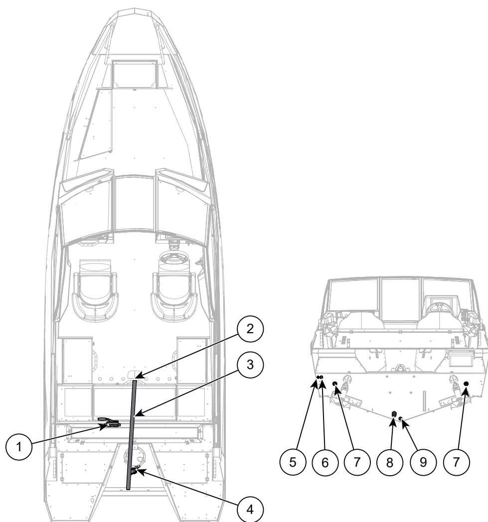
Figur 9.1 Dreneringsutstyr i Buster XL/XXL
