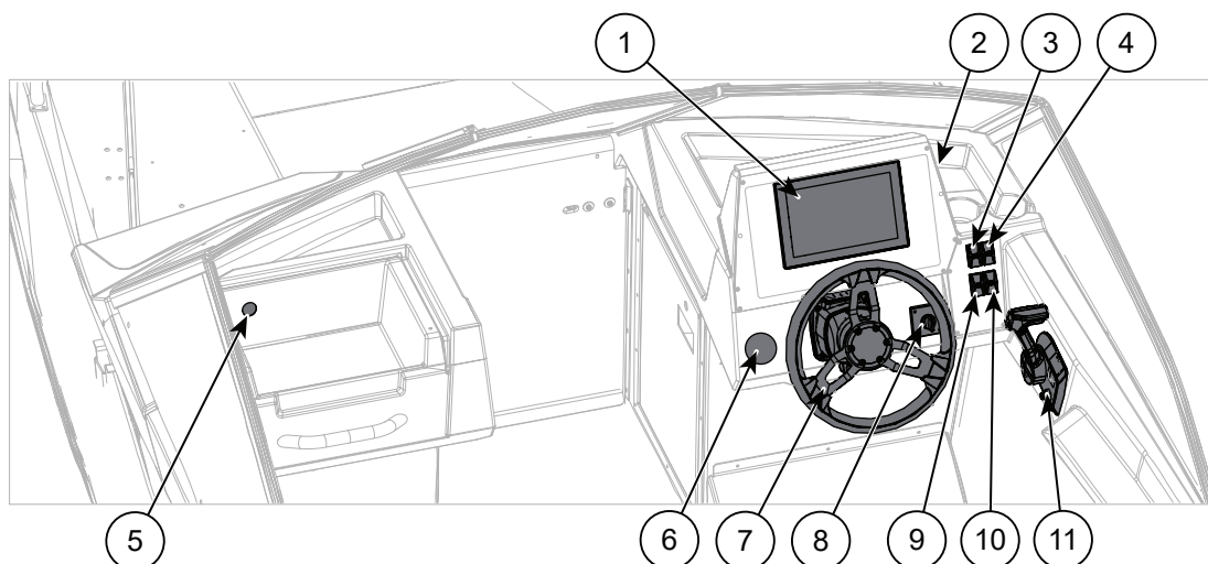
Figur 5.1 Styrestasjonskontroller for Buster XL/XXL
