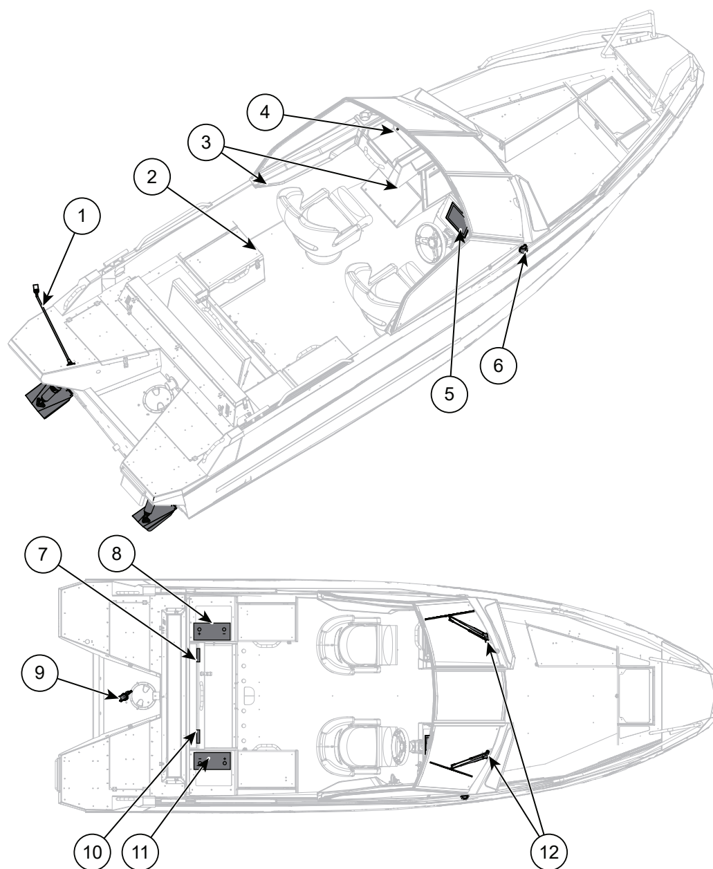
Figur 8.3 Elektrisk utstyr i Buster XL/XXL
