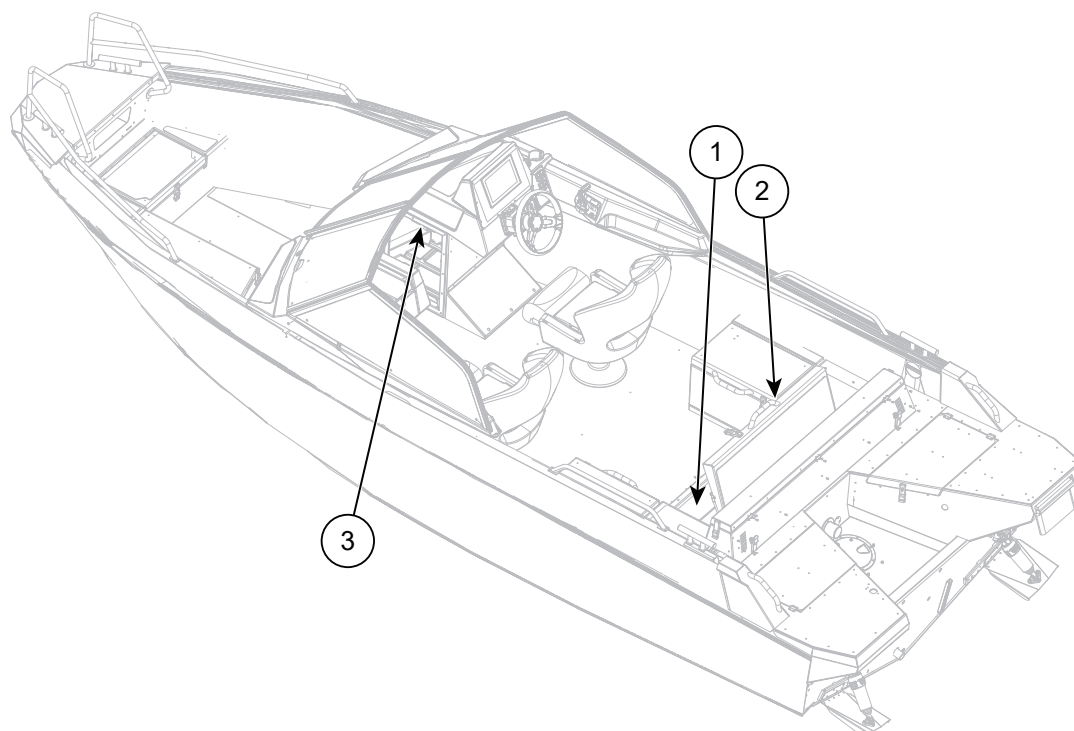
Figur 8.2 Plassering av sikringspaneler i Buster XL/XXL
