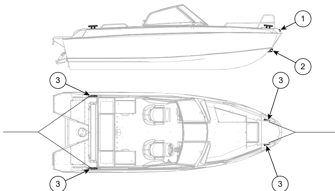
Figur 5.5 Fortøynings- og slepepunkter for Buster XL/XXL
